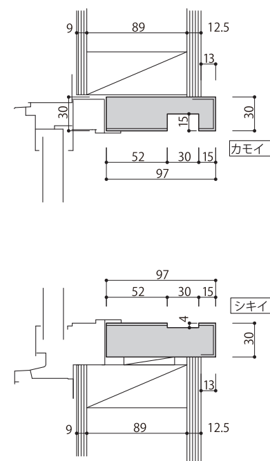
縦断面図
