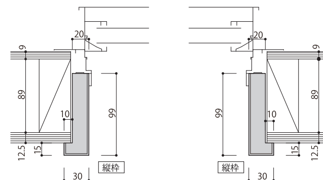
横断面図
