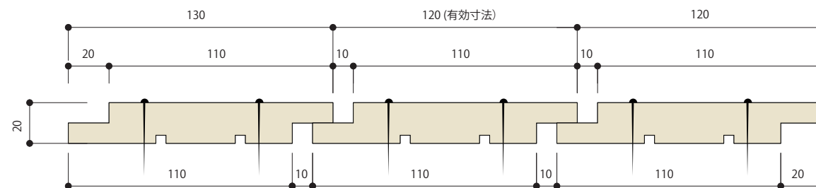
【外壁材 断面図】
