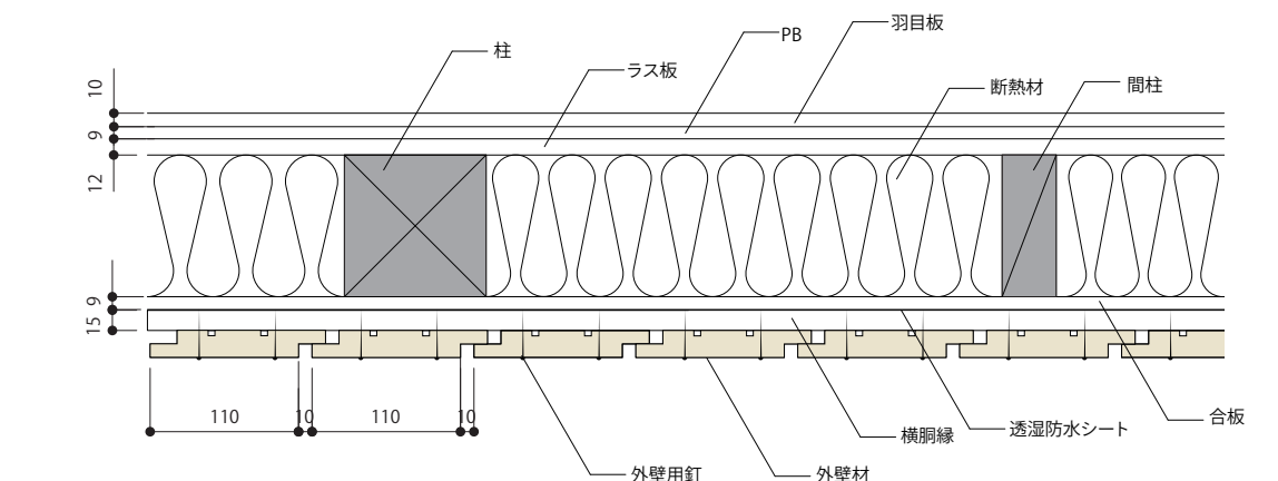
【断面納まり参考図】
