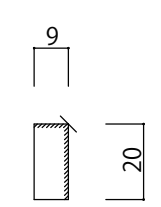
巾木 20×9
