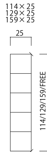
無目枠
