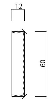
ケーシング 60×12
