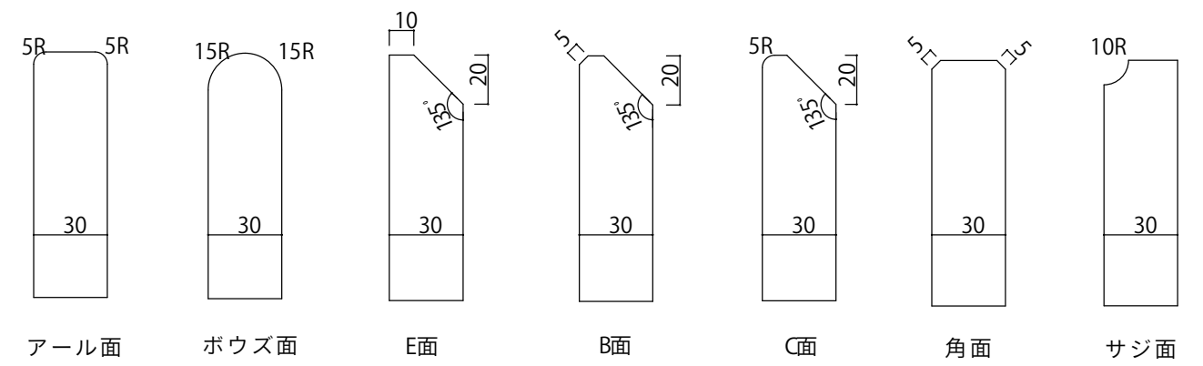
面取り形状
