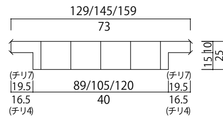
SLIM 笠木
