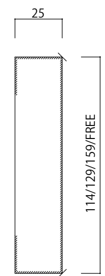
無目枠 114×25 129×25 159×25
