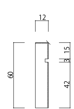
巾木 60×12
