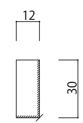
廻り縁 30×12
