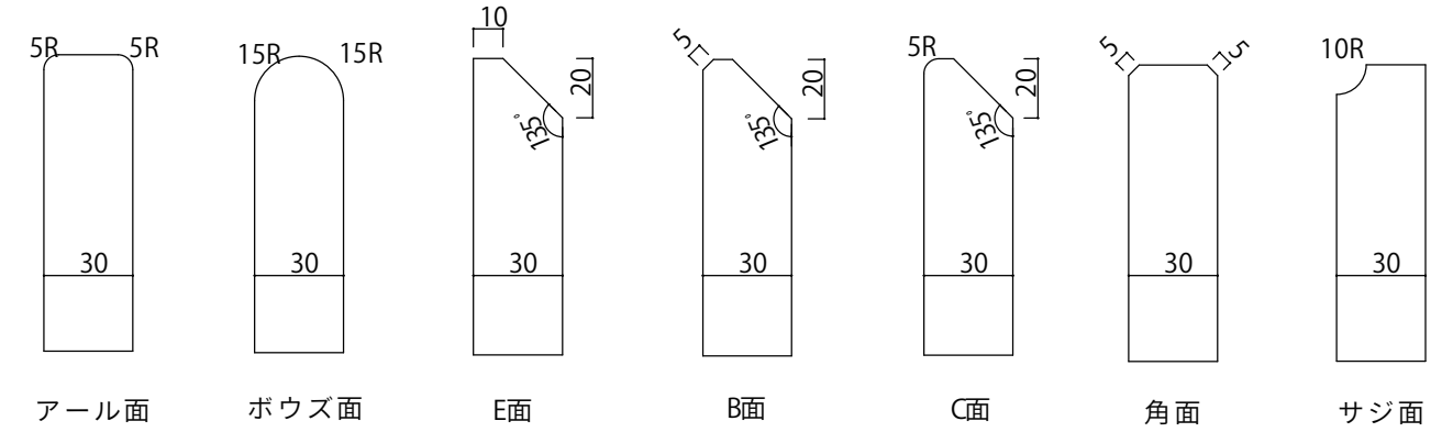
面取り形状
