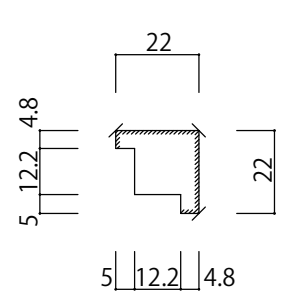
出隅 22×22
