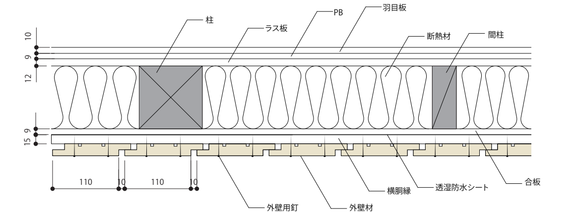
【断面納まり参考図】
