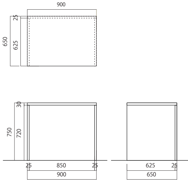
① 〈 W900×D650×H750 〉
