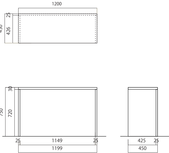
② 〈 W1000×D450×H750 〉
