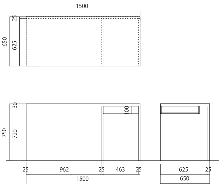
③ 〈 W1500×D650×H750 〉
