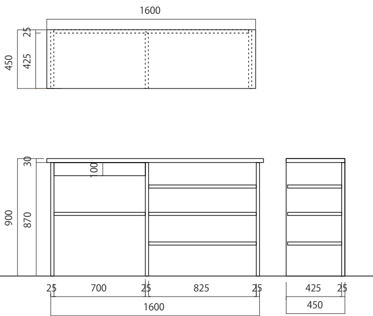
④ 〈 W1600×D450×H900 〉
