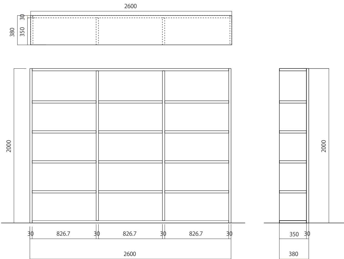
② 〈 W2600×D380×H2000 〉
