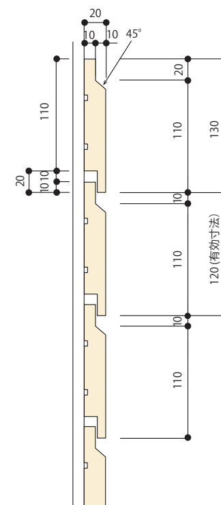
【ボーダー下見板 断面図】
