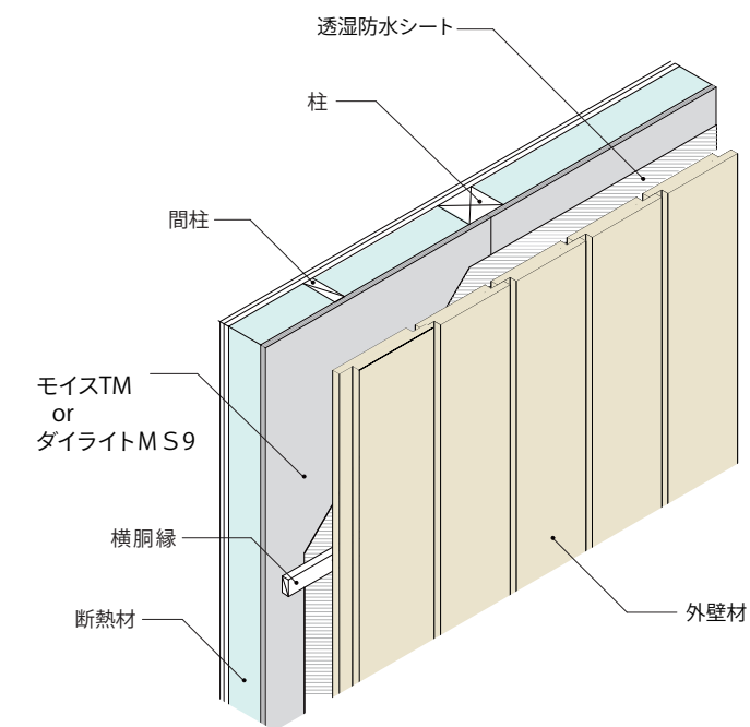
【納まり参考図】
